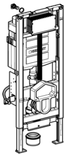
Duofix Wand-WC-Element UP320, Typ 112, Baubreite 42.5 cm
