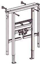
Duofix Element für Waschtisch mit Unterputz-Sifon, Typ 112, ausziehbar
